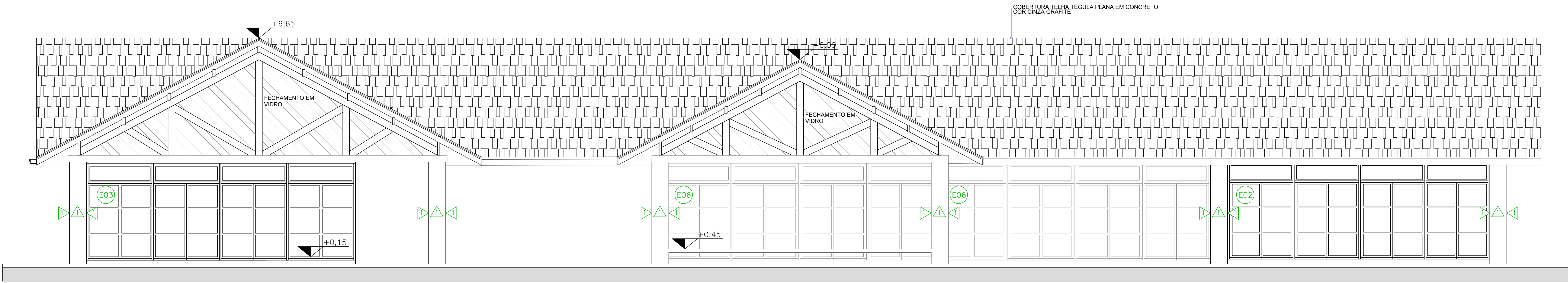
ELEVAÇÃO 3 ESCALA 1:50
