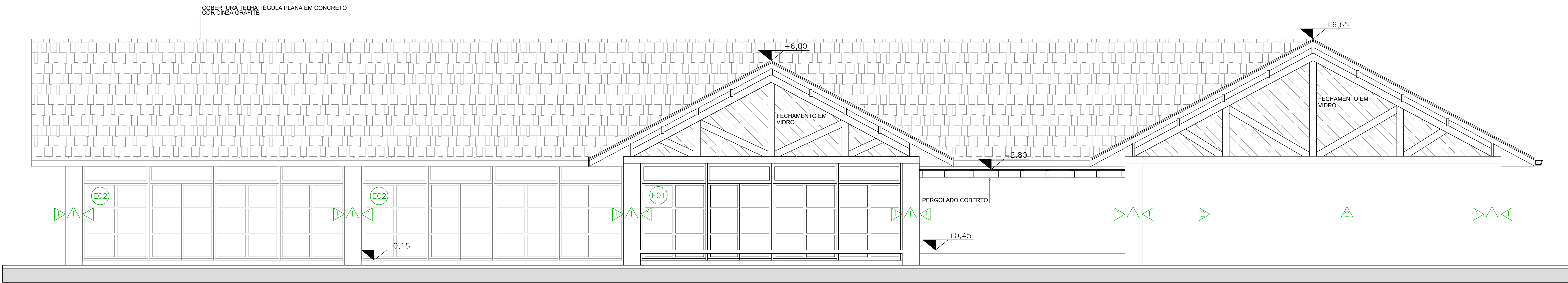
ELEVAÇÃO 1 ESCALA 1:50
