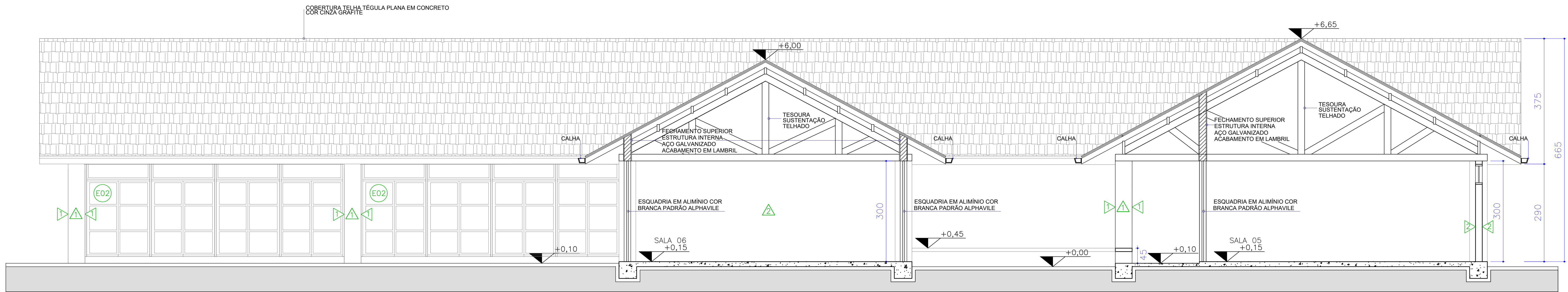
CORTE AA ESCALA 1:50
