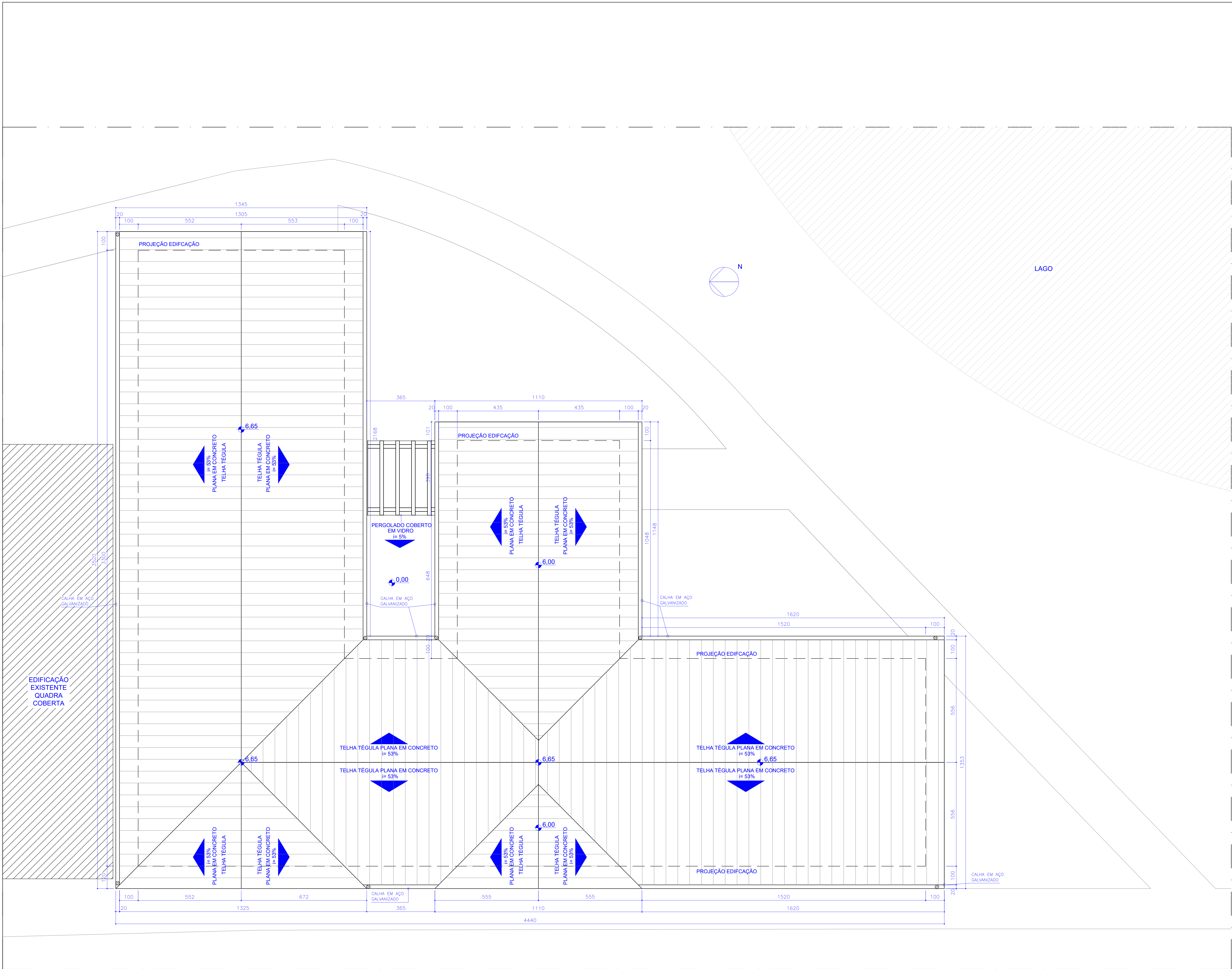
PLANTA DE COBERTURA ESCALA 1:75
