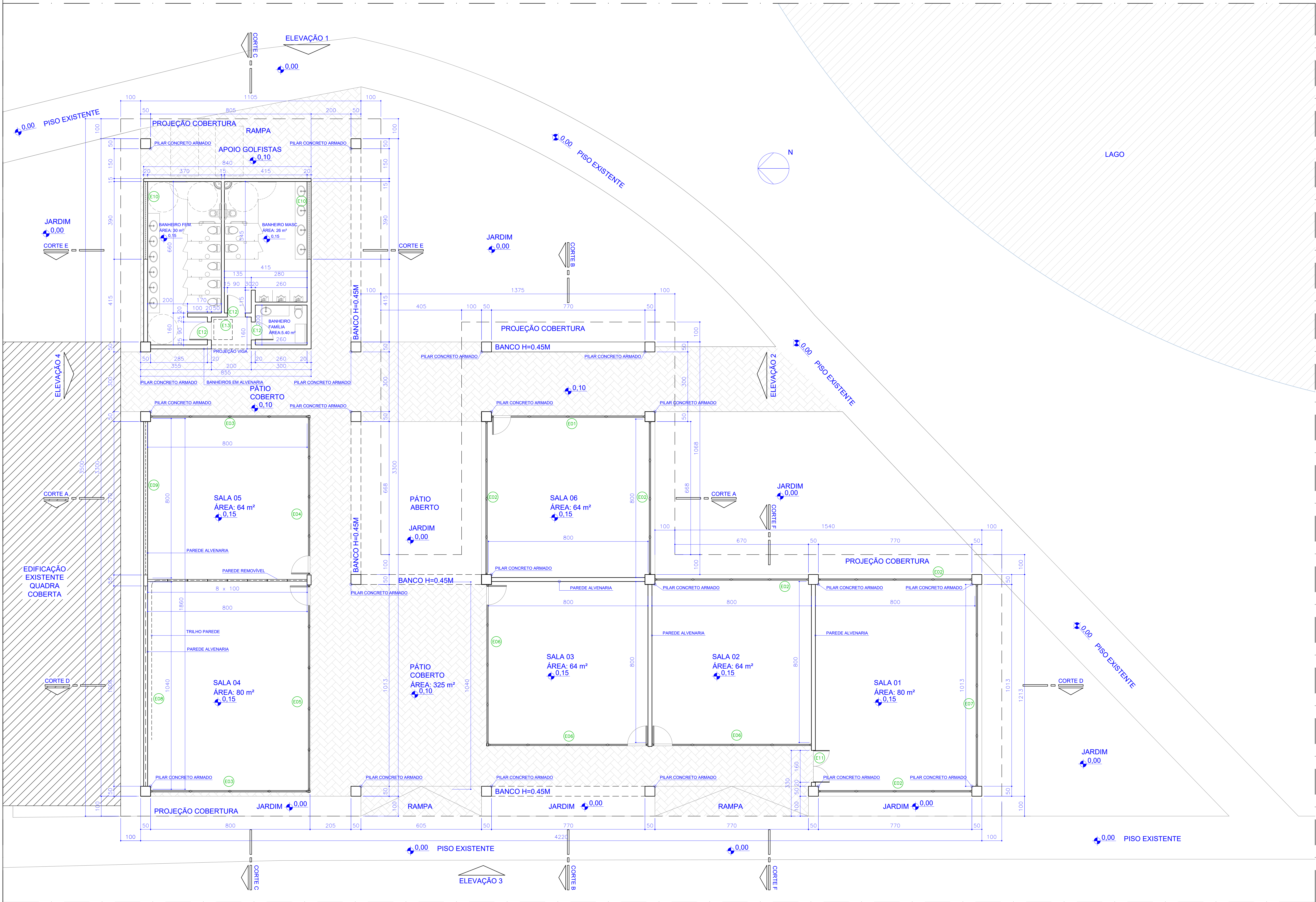
PLANTA PAV. TÉRREO ESCALA 1:75
