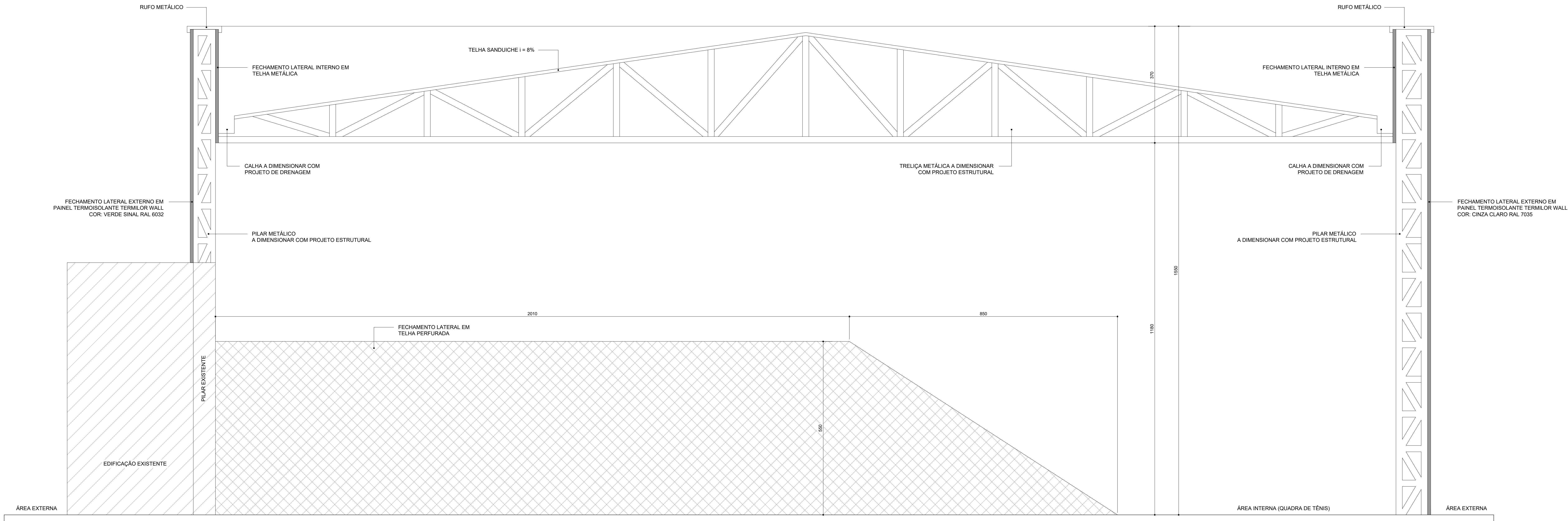
CORTA A-A ESCALA 1:50
