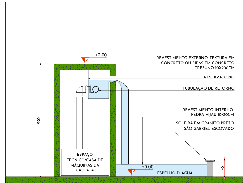
DET 5. CASCATA
