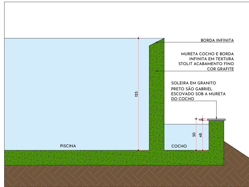
DET 3. BORDA INFINITA
