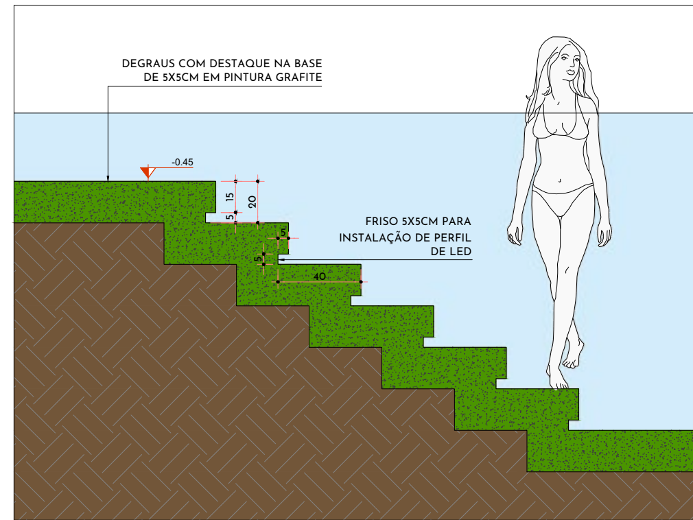
DET 4. ESCADA
