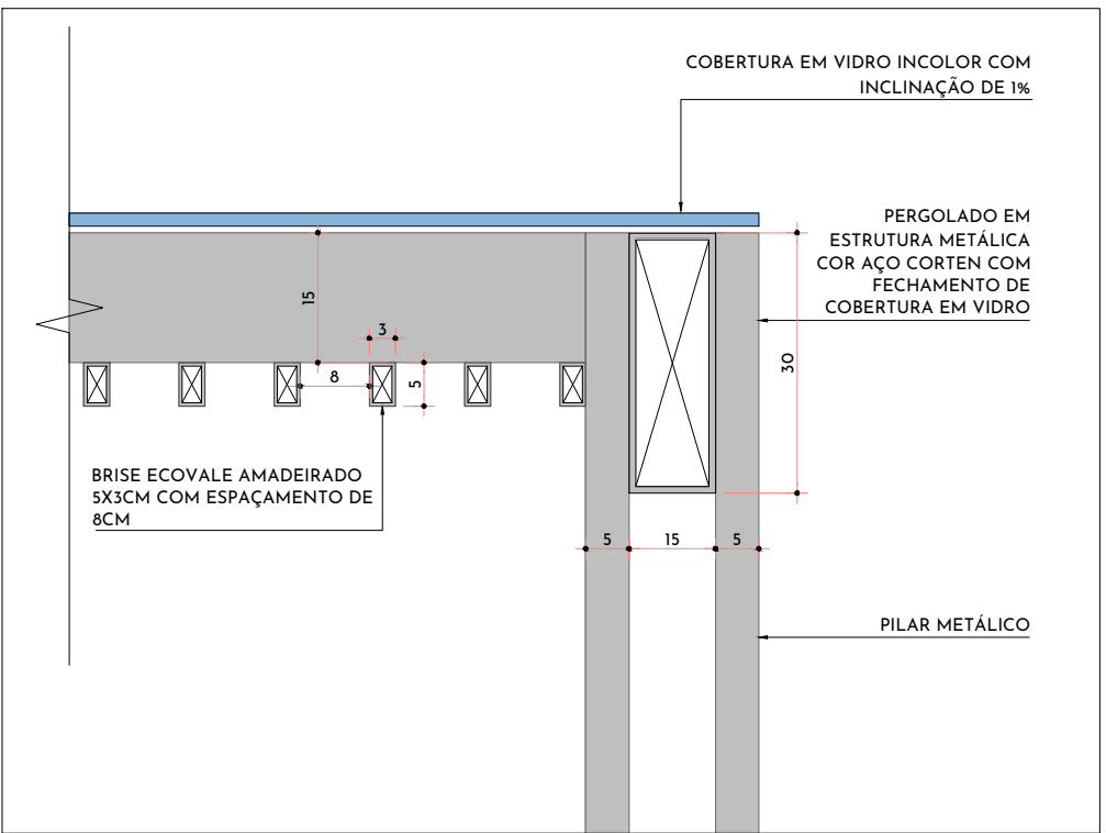
DET 1. PERGOLADO
