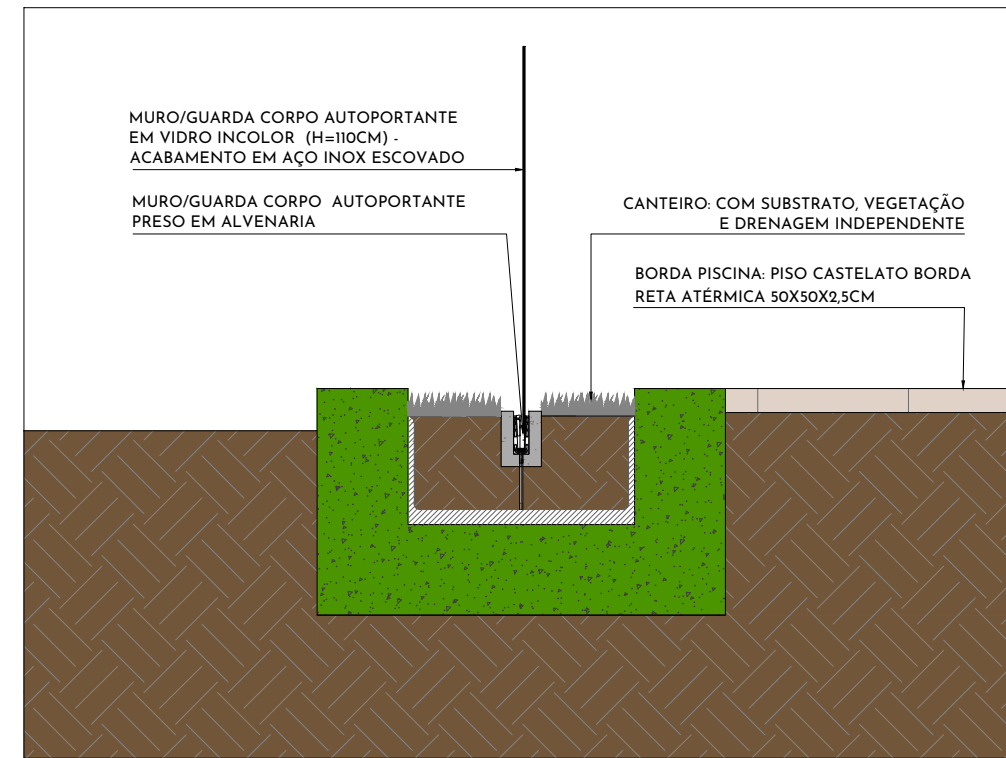
DET 6. FLOREIRA + GUARDA CORPO
