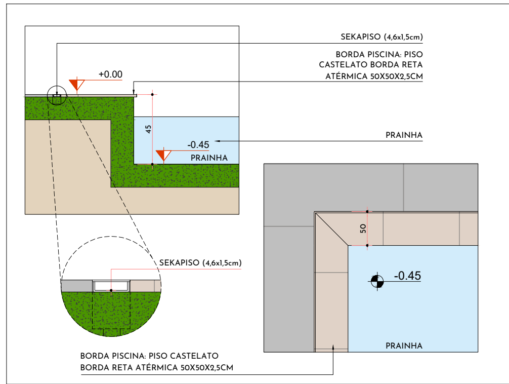
DET 2. BORDA PISCINA
